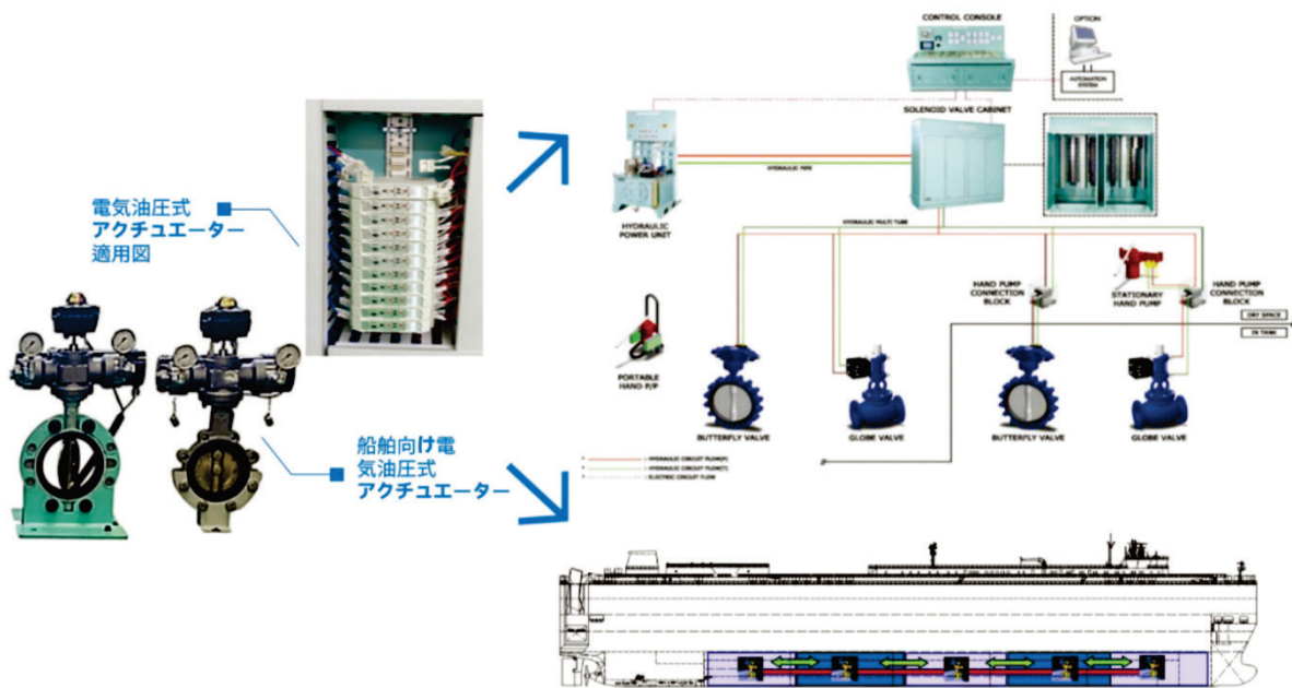
<電気油圧式アクチュエーター適用図>
